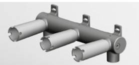
Parte empotrada con cuerpo unico, distancia entre eje de 200 mm.
