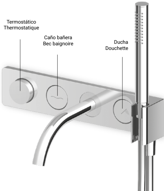
ZHO825+R96706 Termostático baño-ducha empotrado Thermostatique bain-douche à encastrer
